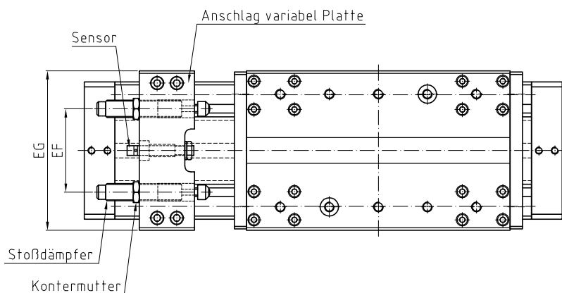
Maßtabelle
